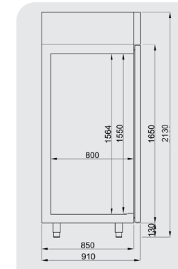
Ölçü Detayları Dimension Details
