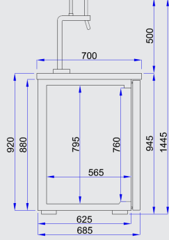
Ölçü Detayları Dimension Details
